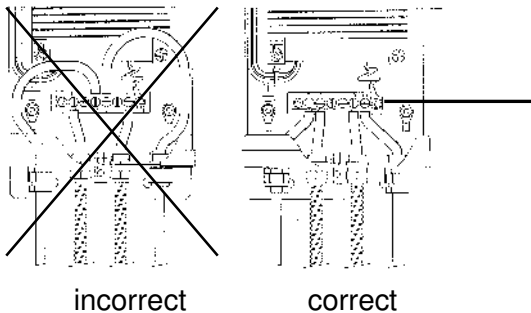
Illustration 3: Connexion des câbles dans l'alimentation
