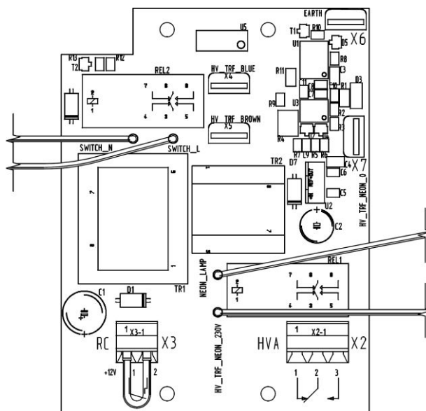
Abbildung 11: Optionale HRD-Leiterplatte
